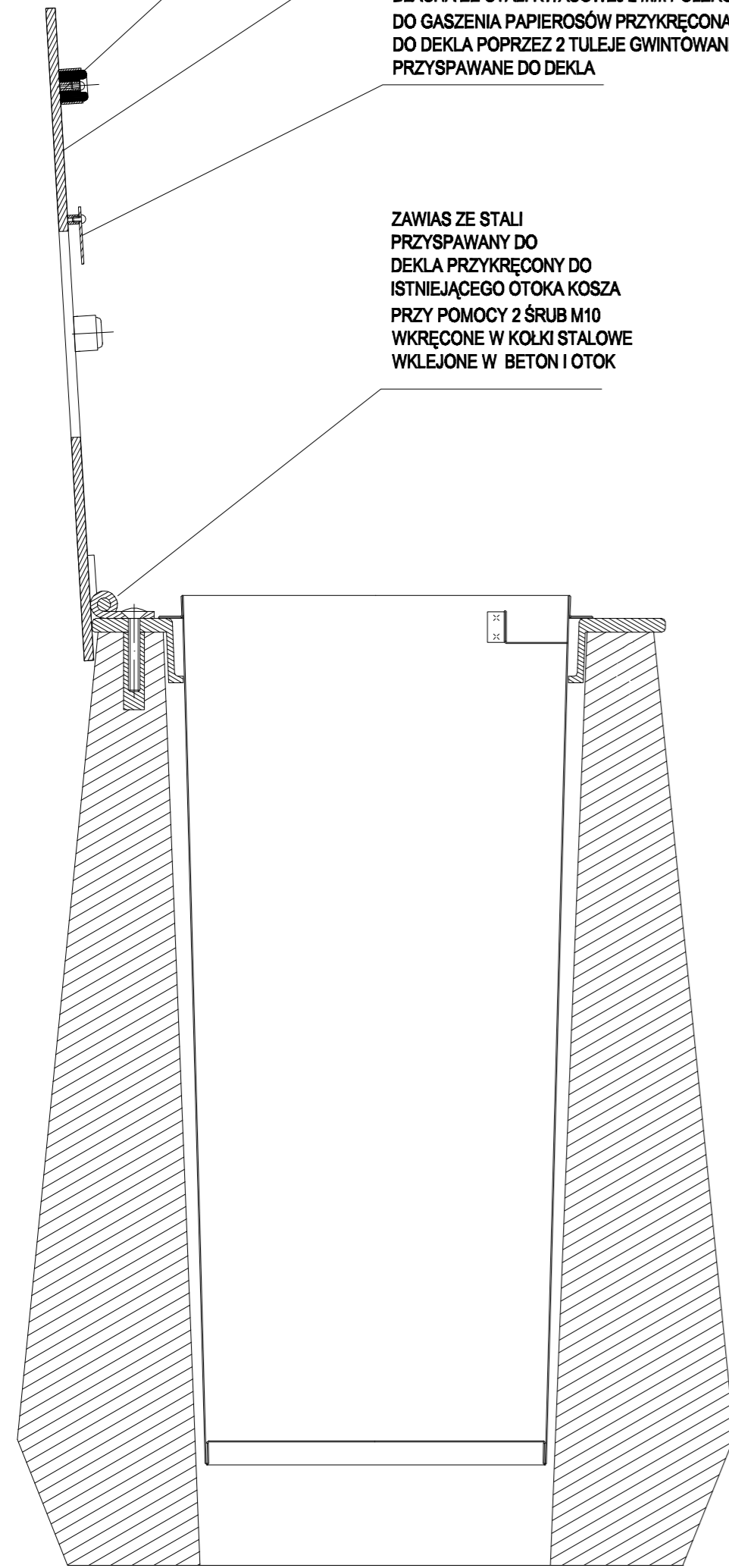
PRZEKRÓJ AA Z ODCHYŁONYM DEKLEM SKALA 1:5
